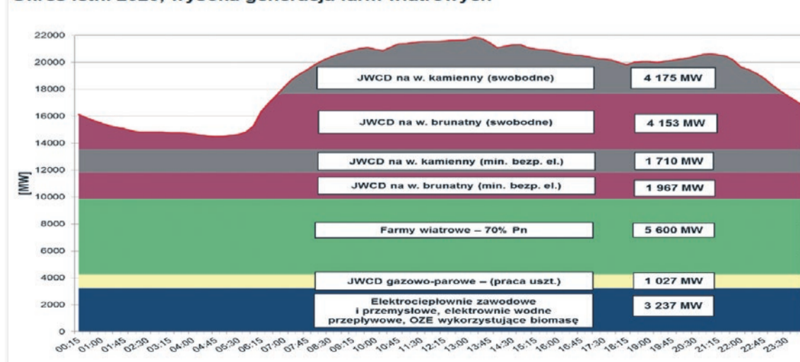
Okres letni 2020, wysoka generacja farm wiatrowych
